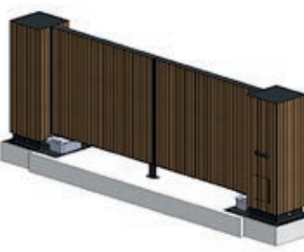
Modell C - King Standardhöhe: 1800 mm Standardbreiten: 3500 | 4000 mm Aluminium Pfosten ohne Verkleidung (500 x 500 mm) - wahlweise mit Holzverkleidung (580 x 580 mm), mit oder ohne integriertem Paketbriefkasten
