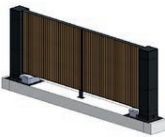
Modell B - Queen Standardhöhe: 1800 mm Standardbreiten: 3800 | 4300 | 4800 mm Aluminium Pfosten ohne Verkleidung (320 x 320 mm) - wahlweise mit Holzverkleidung (400 x 400 mm), mit oder ohne integriertem Paketbriefkasten
