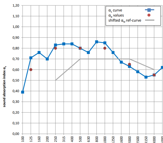
Gemiddelde geluidsabsorptie bij plenumhoogte 250 mm
