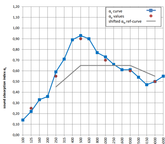
Gemiddelde geluidsabsorptie bij plenumhoogte 50 mm
