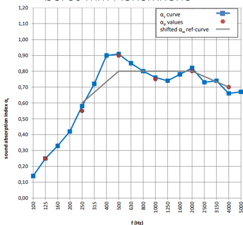
Durchschnittliche Schallabsorption bei 50 mm Plenumhöhe
