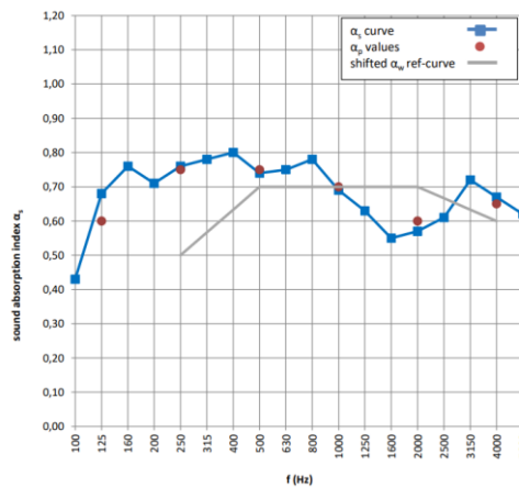
Durchschnittliche Schallabsorption bei 250 mm Plenumhöhe
