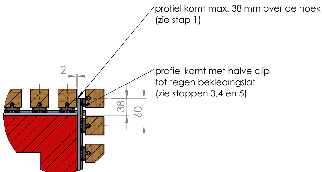
DETAIL A schaal 1 : 5
