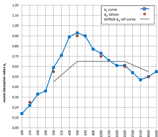
Absorption acoustique moyenne avec une hauteur plénum de 50 mm
