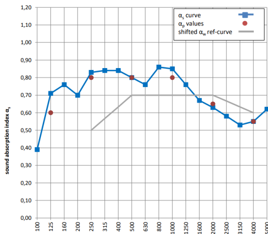
Absorption acoustique moyenne avec une hauteur plénum de 250 mm
